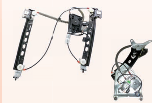
LÈVE - VITRES POWER WINDOW
